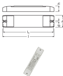
Scheda tecnica Osram LED Driver OPTOTRONIC Intelligent Dali UNV1 240V 1-4CH | Dimmerabile
